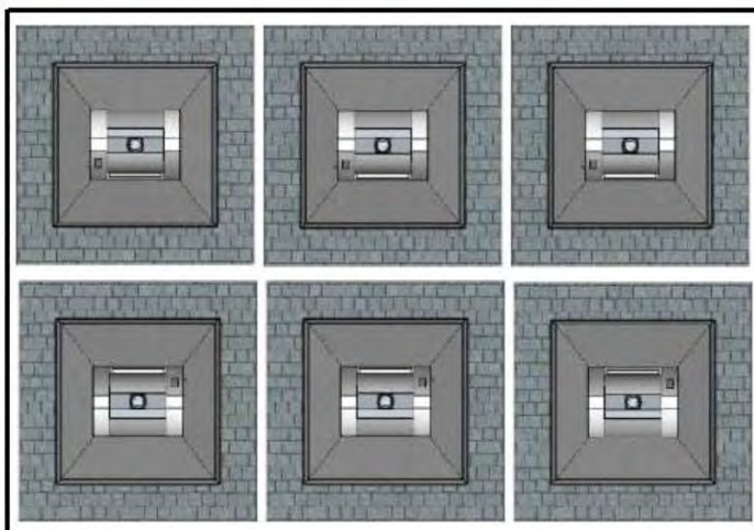
Exemple pose par 4 ou 6 conteneurs en opposition
