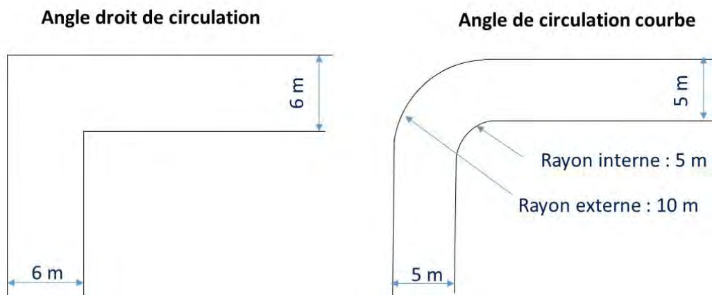
Figure 1 : Virage possible des véhicules de collecte
