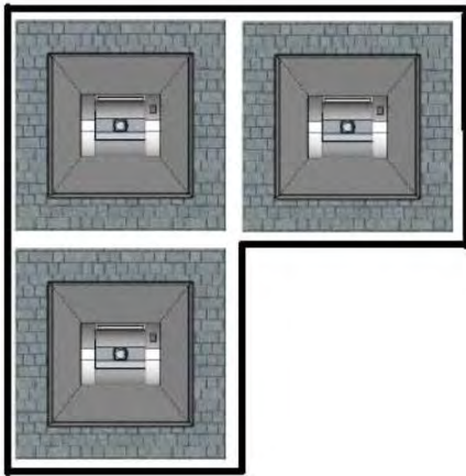
Exemple pose par 3 en L (ouverture vers l'extérieur)
