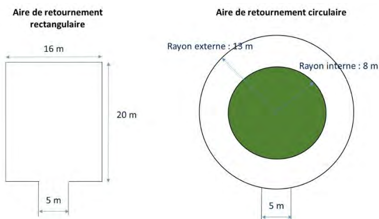
Figure 2 : Dimensionnement des aires de retournement
